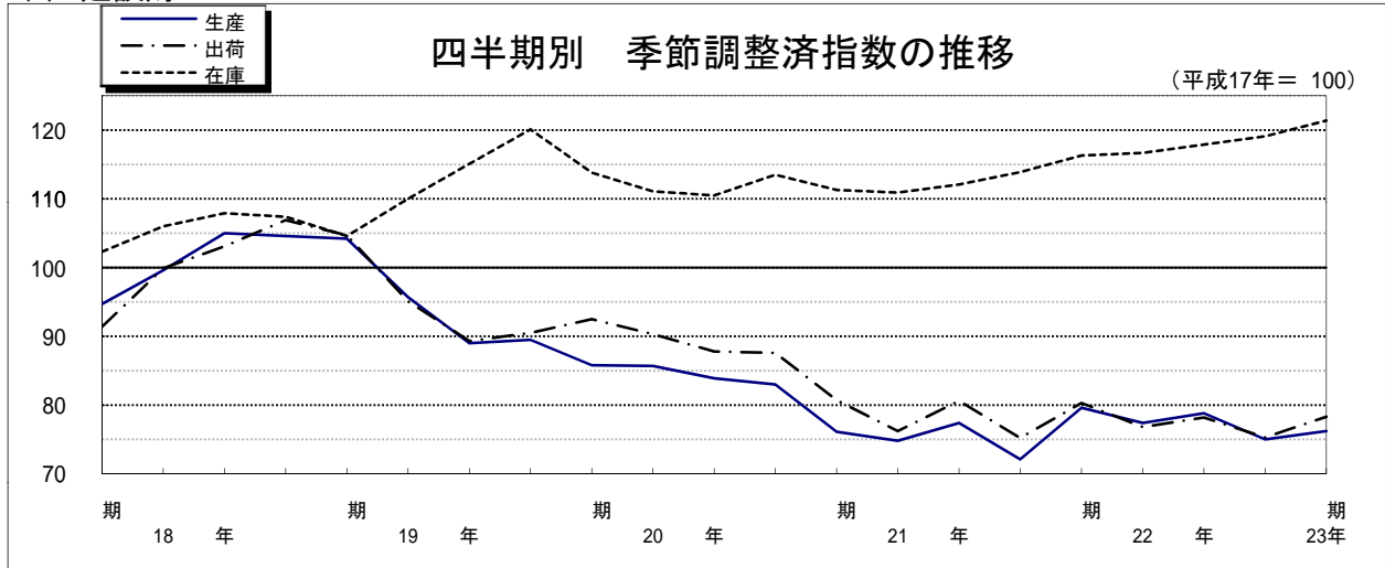
建設財 年別・四半期別指数の推移 (平成17年 = 100)
