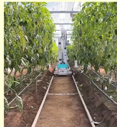
〈ピーマン自動収穫ロボット〉
