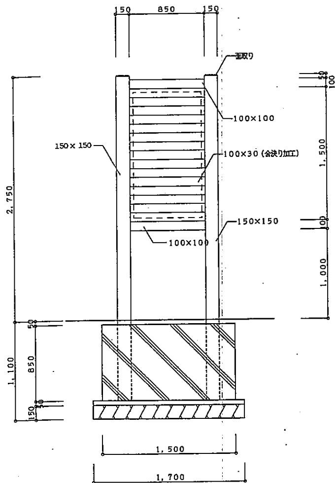
立面図 S=1/30
