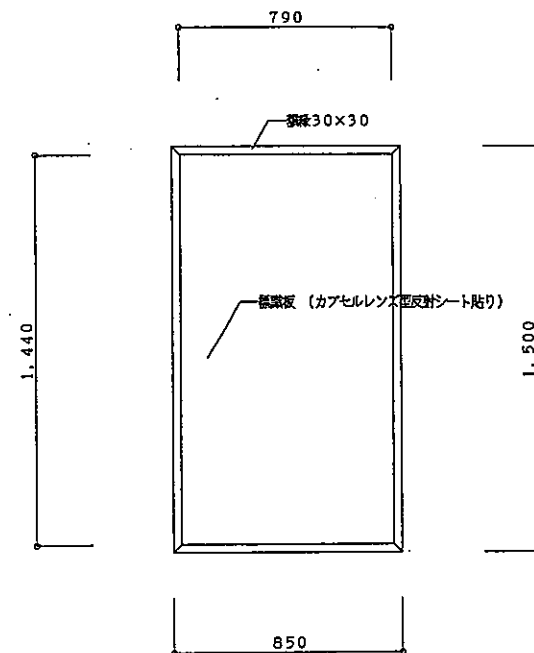
標識板詳細図 S=1/20
