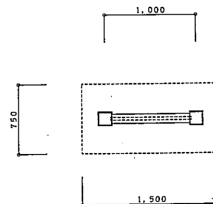
標識板詳細図 S=1/20
