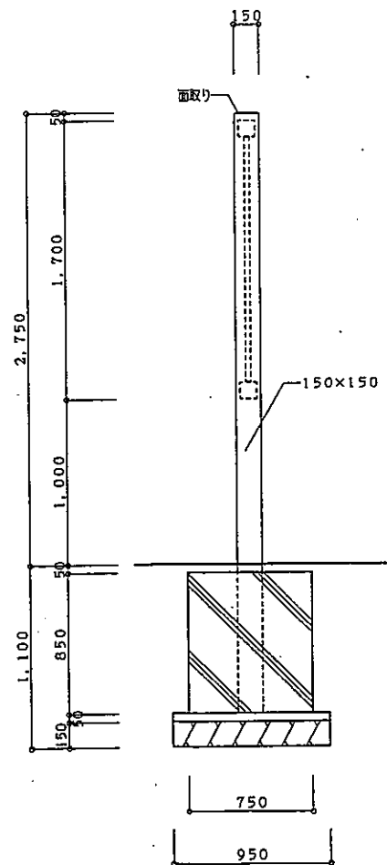
立面図 S=1/30
