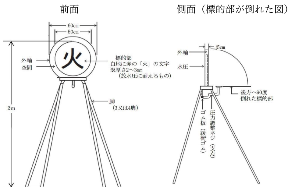
(別図) 有効放水測定装置付標的
