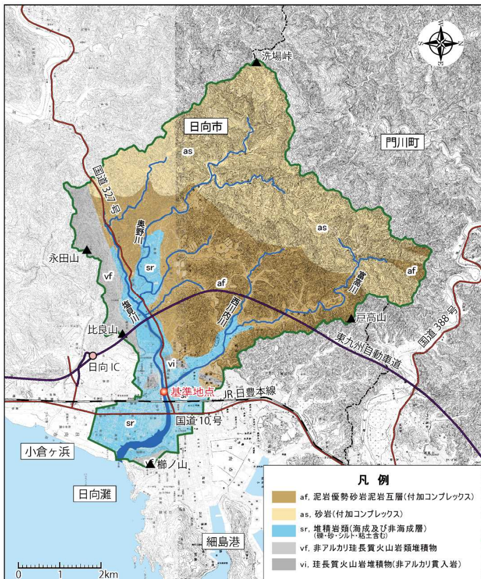
図 1-2 流域の地質図
