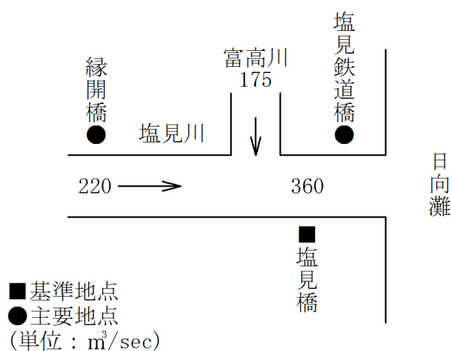
図 4-1 塩見川における整備計画の対象流量
