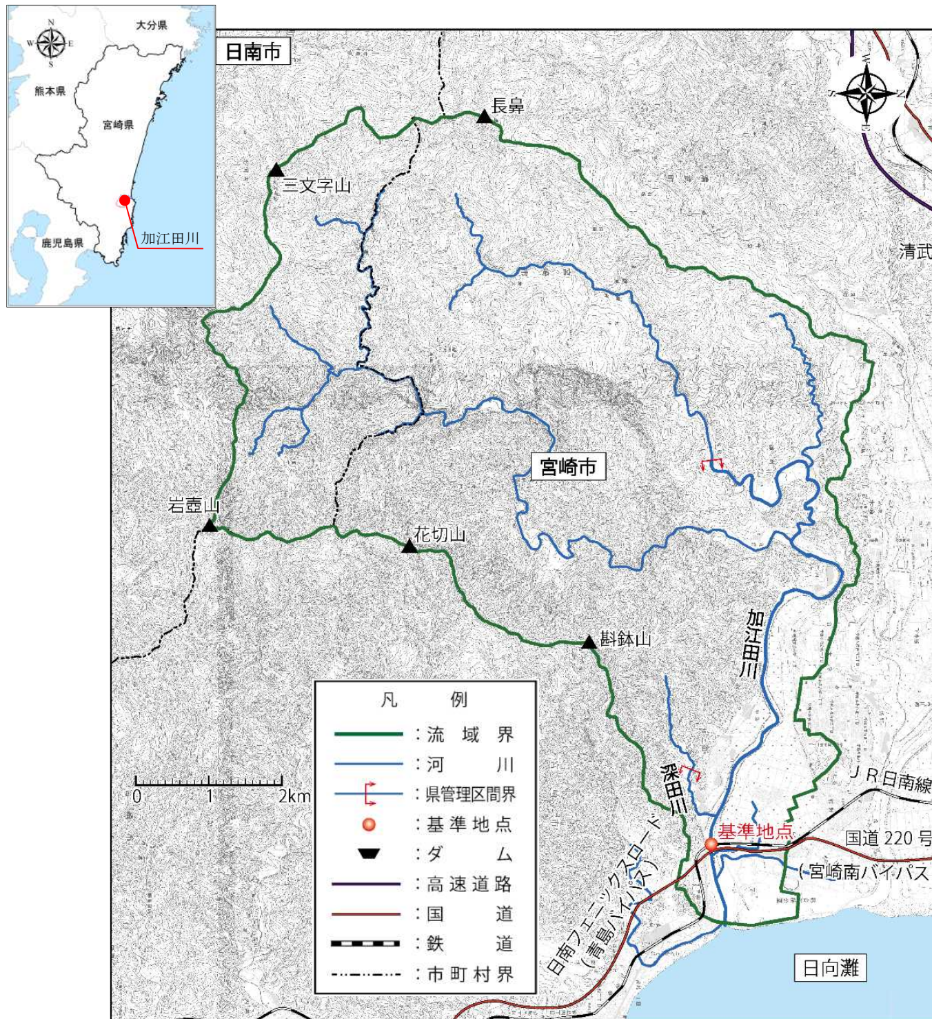
(参考図) 加江田川水系図
