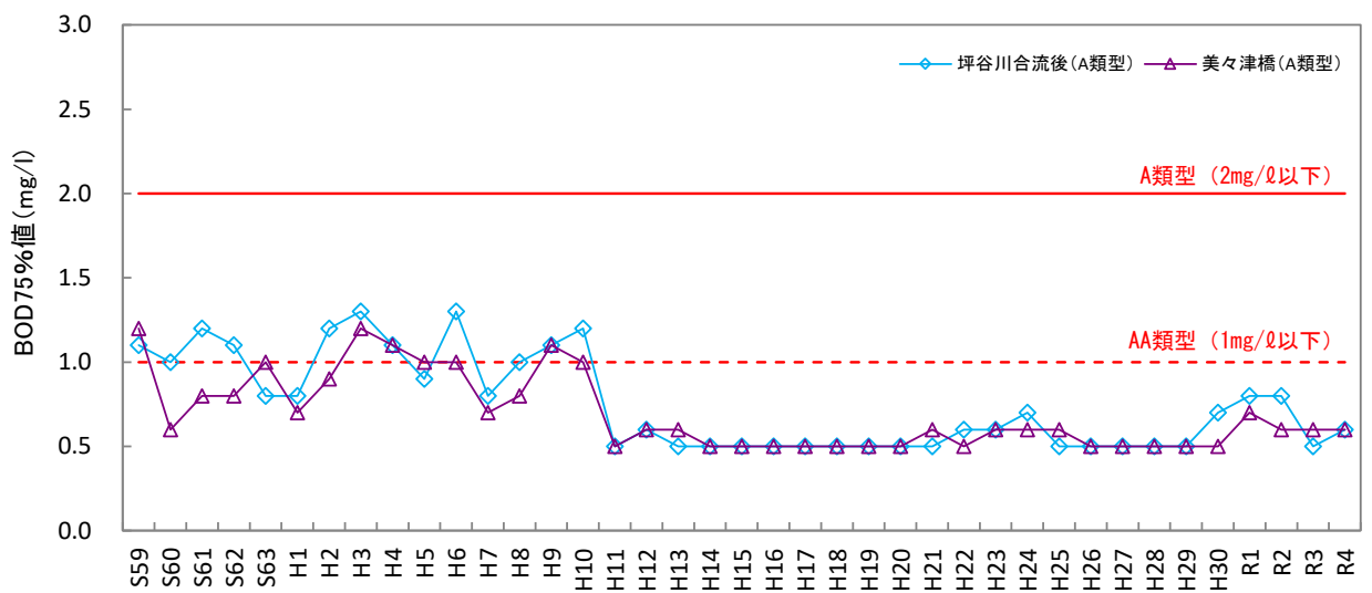
図-2 主要地点における水質(BOD75%値)の経年変化
