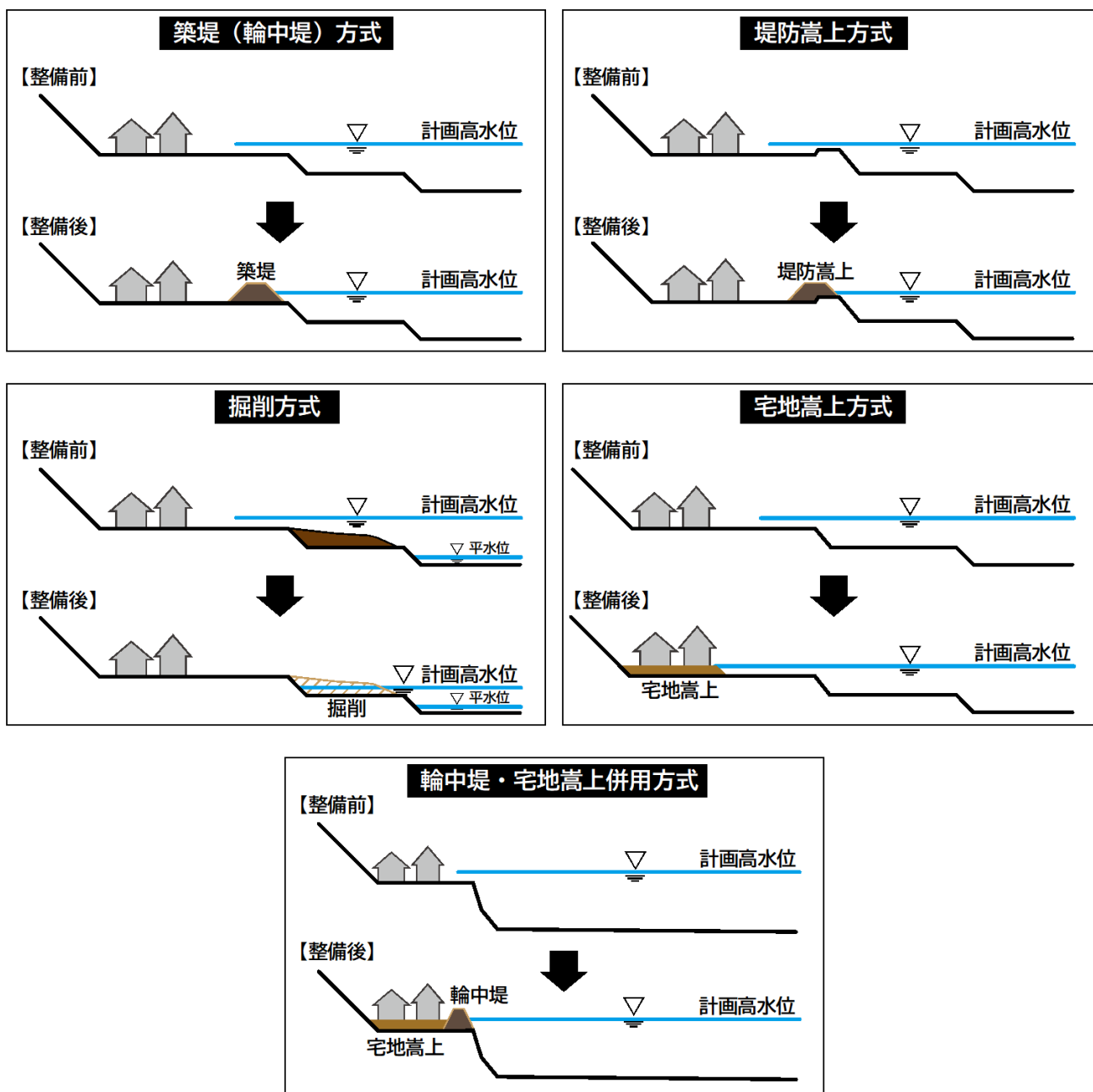
図－9 治水対策方式のイメージ図
