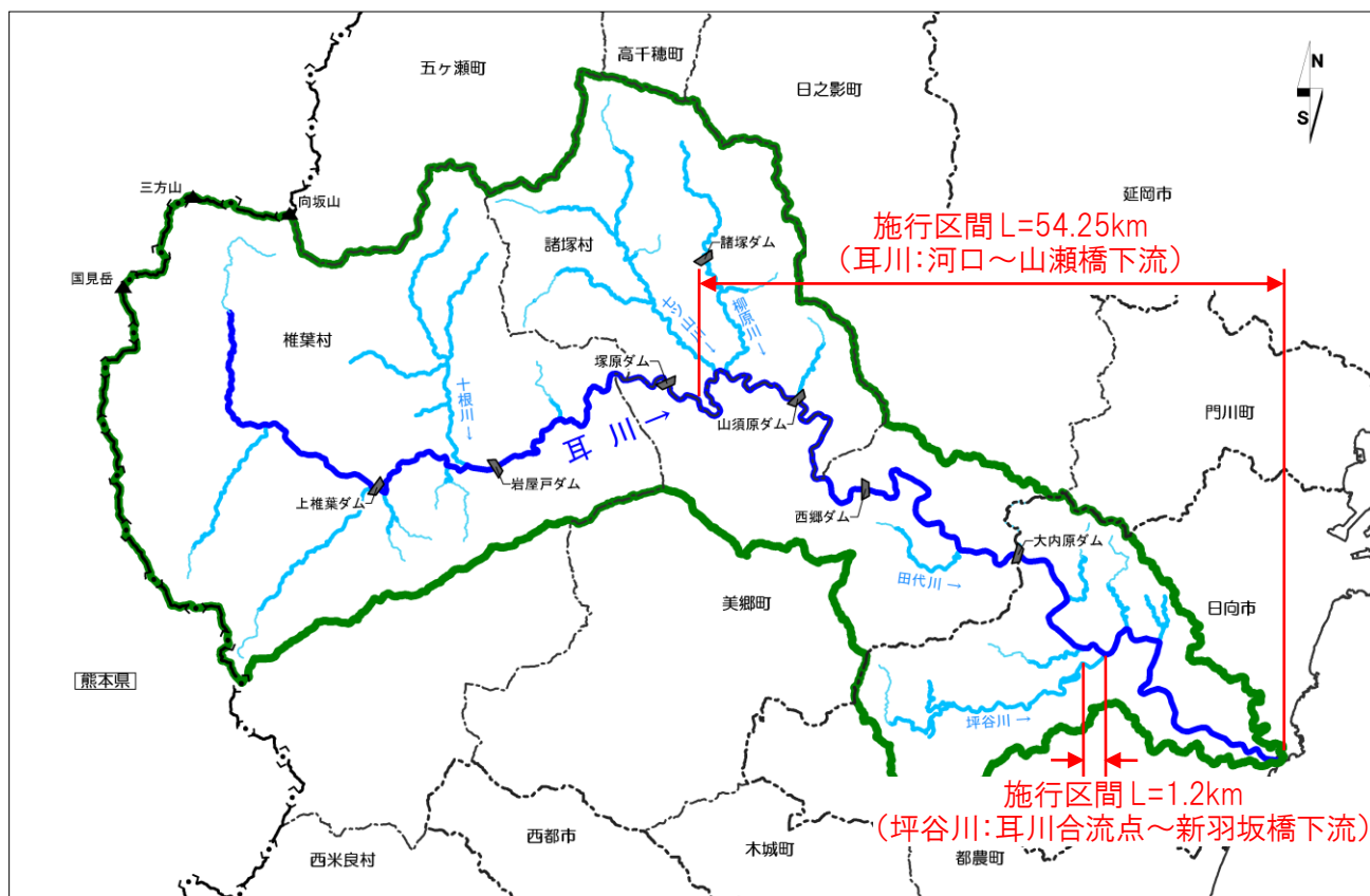
図一5 施行区間(全体図:赤表記)
