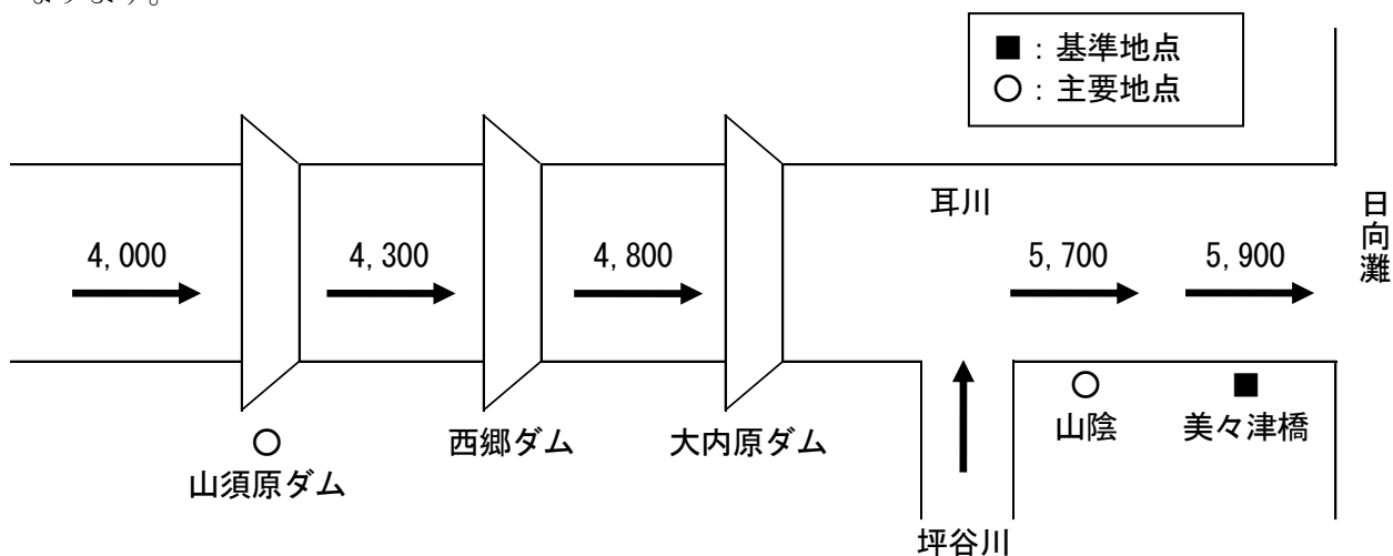
図-4 計画高水流量配分図(単位:m³/s)
