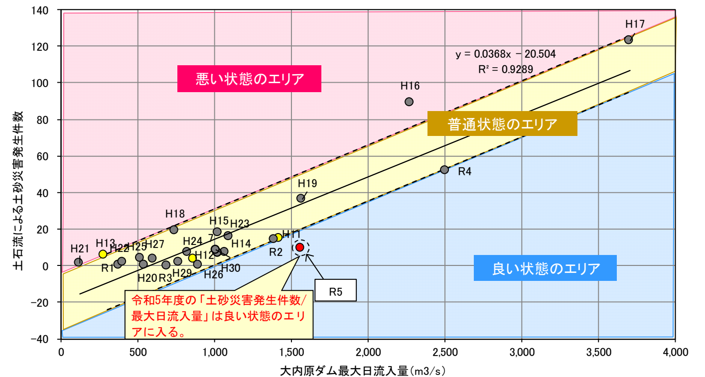
図2-5 土砂災害発生件数と大内原ダム最大日流入量の相関図
