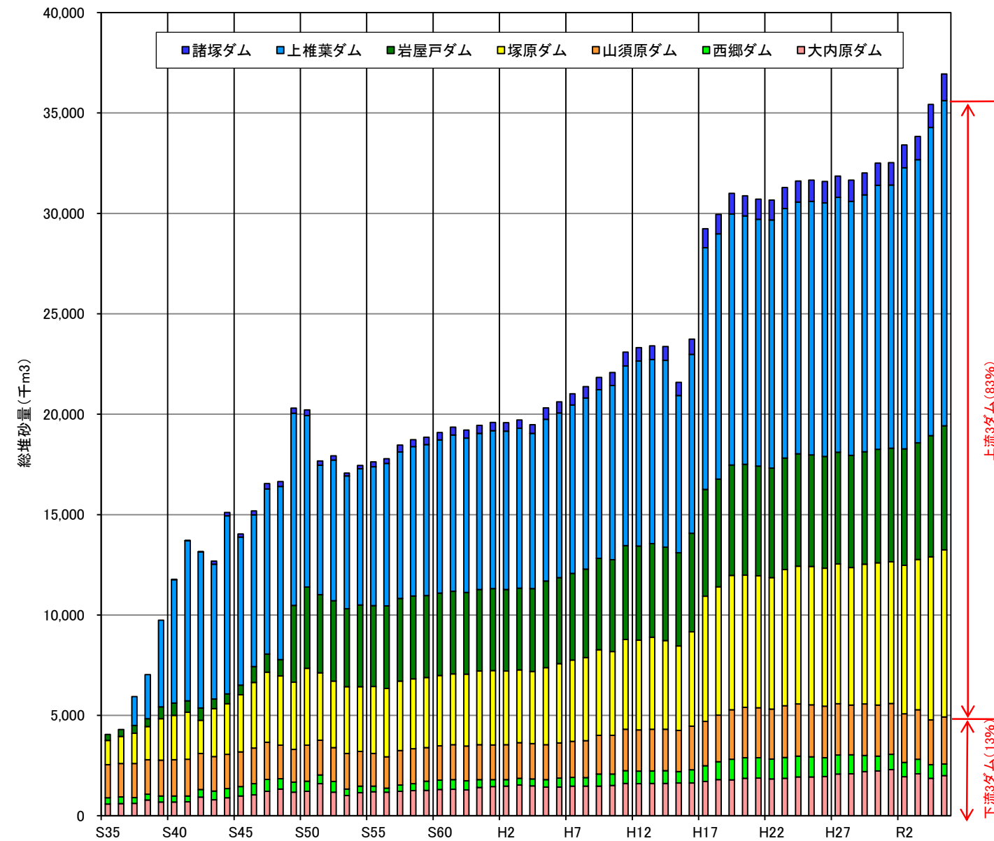
図1-6 ダム堆砂量の経年変化
