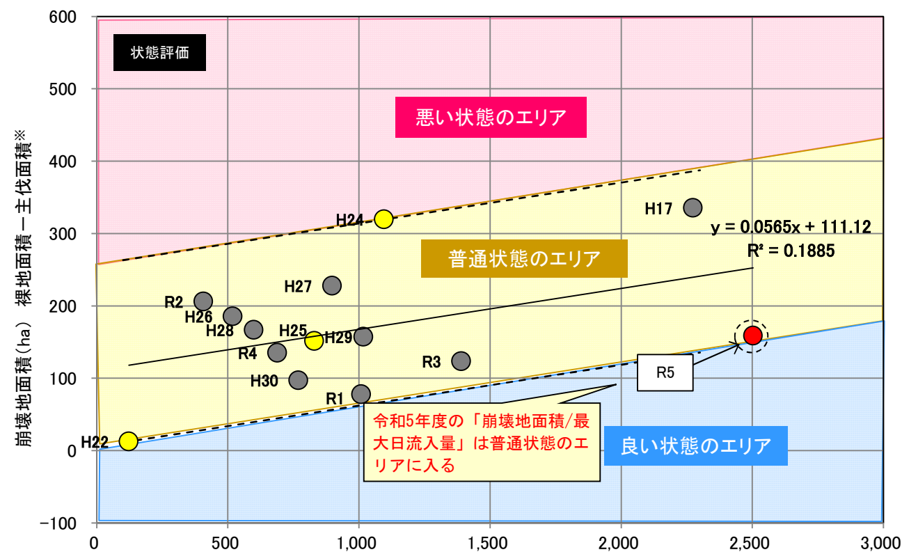
大内原ダム最大日流入量※(m 3 /s) ※前年データ 図5-3 崩壊地面積と大内原ダム最大日流量の相関図
