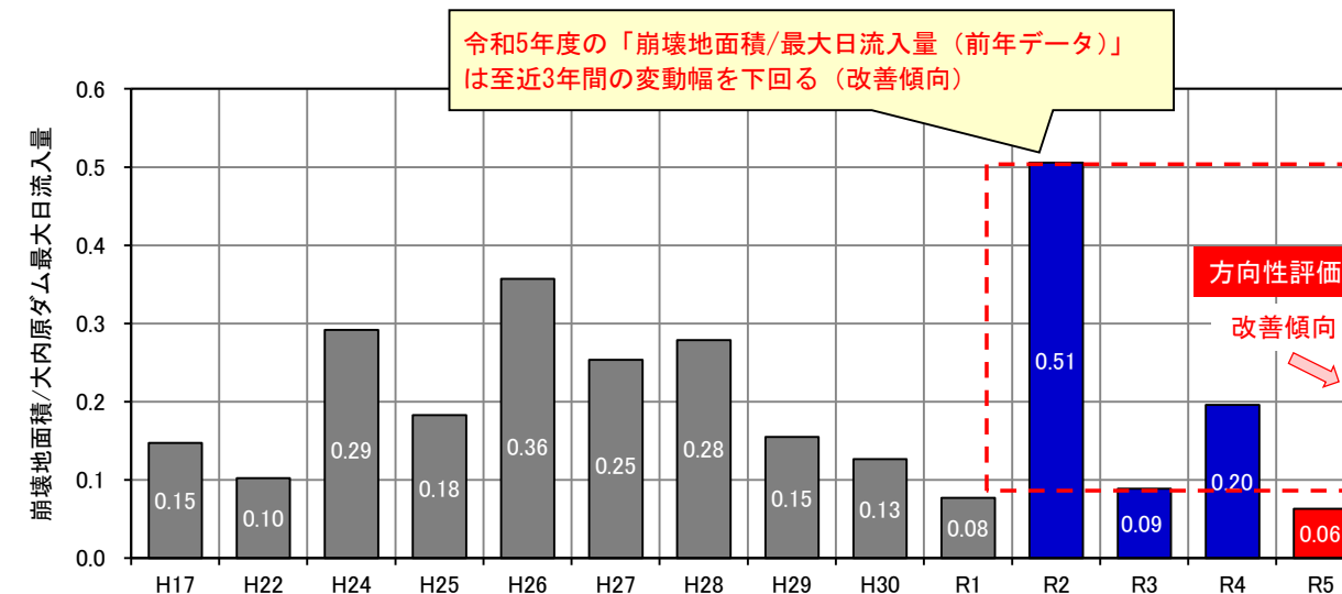
図5-2 崩壊地面積/大内原ダム最大日流入量の経年変化
