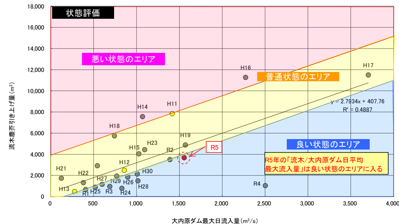
図5-6 流木塵芥引き上げ量/日平均最大流入量の相関図（状態評価）
