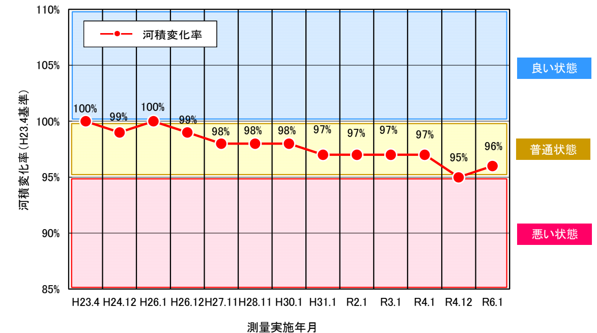
図1-10 河積変化率の経年変化
