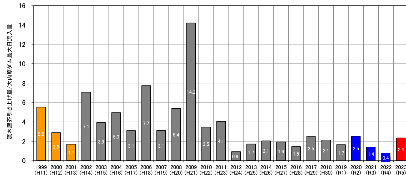
図5-5 流木塵芥引き上げ量/大内原ダム最大日流入量の経年変化
