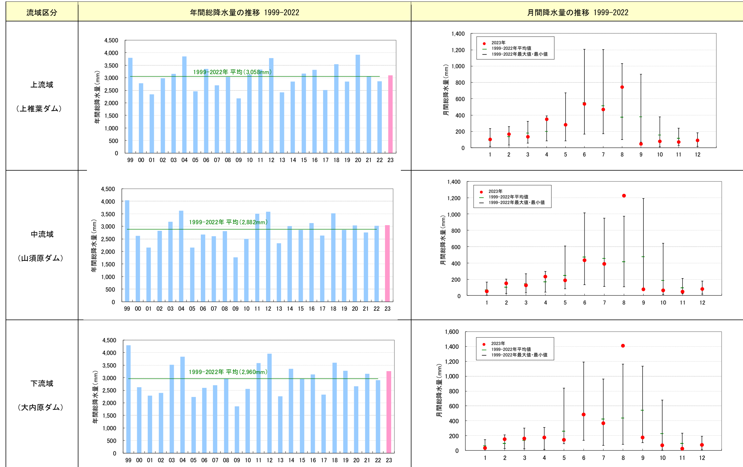
図6-2 耳川流域における降水量の推移 1999-2023（平成11年～令和5年）
