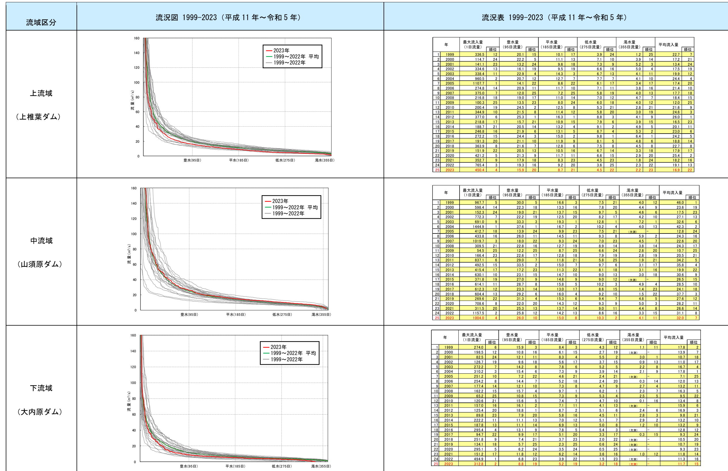
図6-3 耳川流域における流況図及び流況表 1999～2023（平成11年～令和5年）
