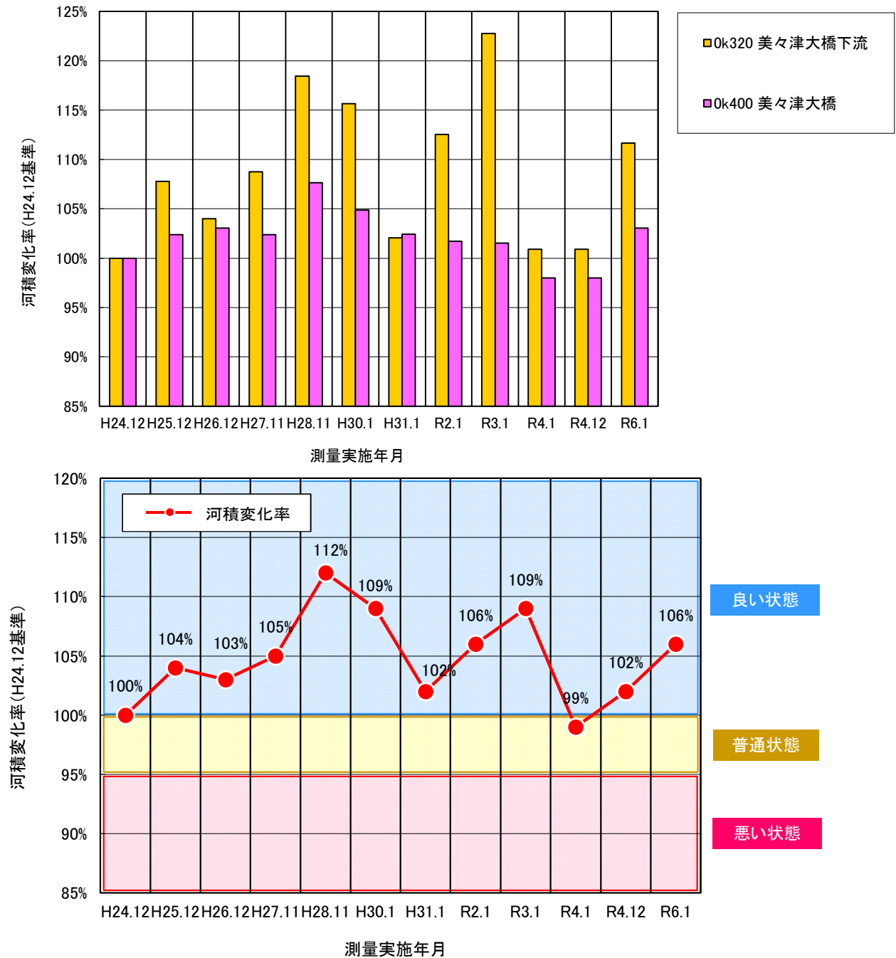
図29-1 河積変化率の経年変化
