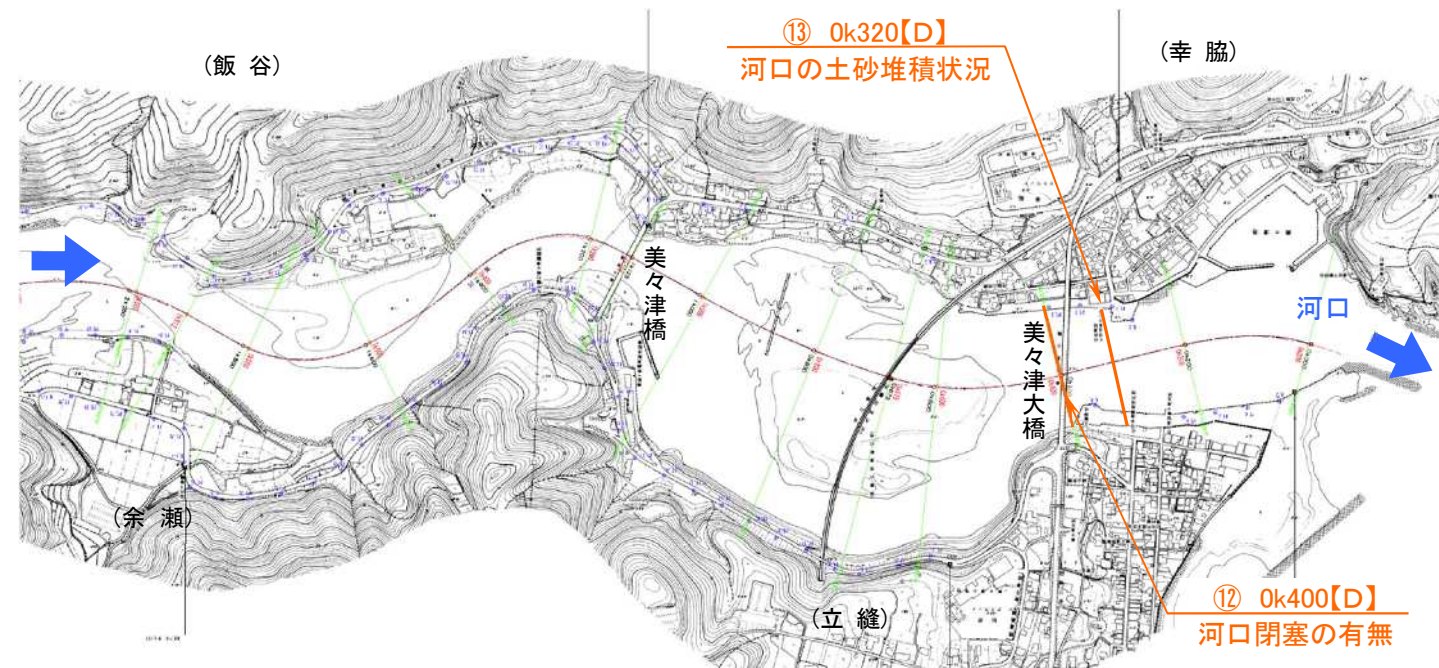
図 29-3 美々津大橋下流（Ok320）の河道横断地形
