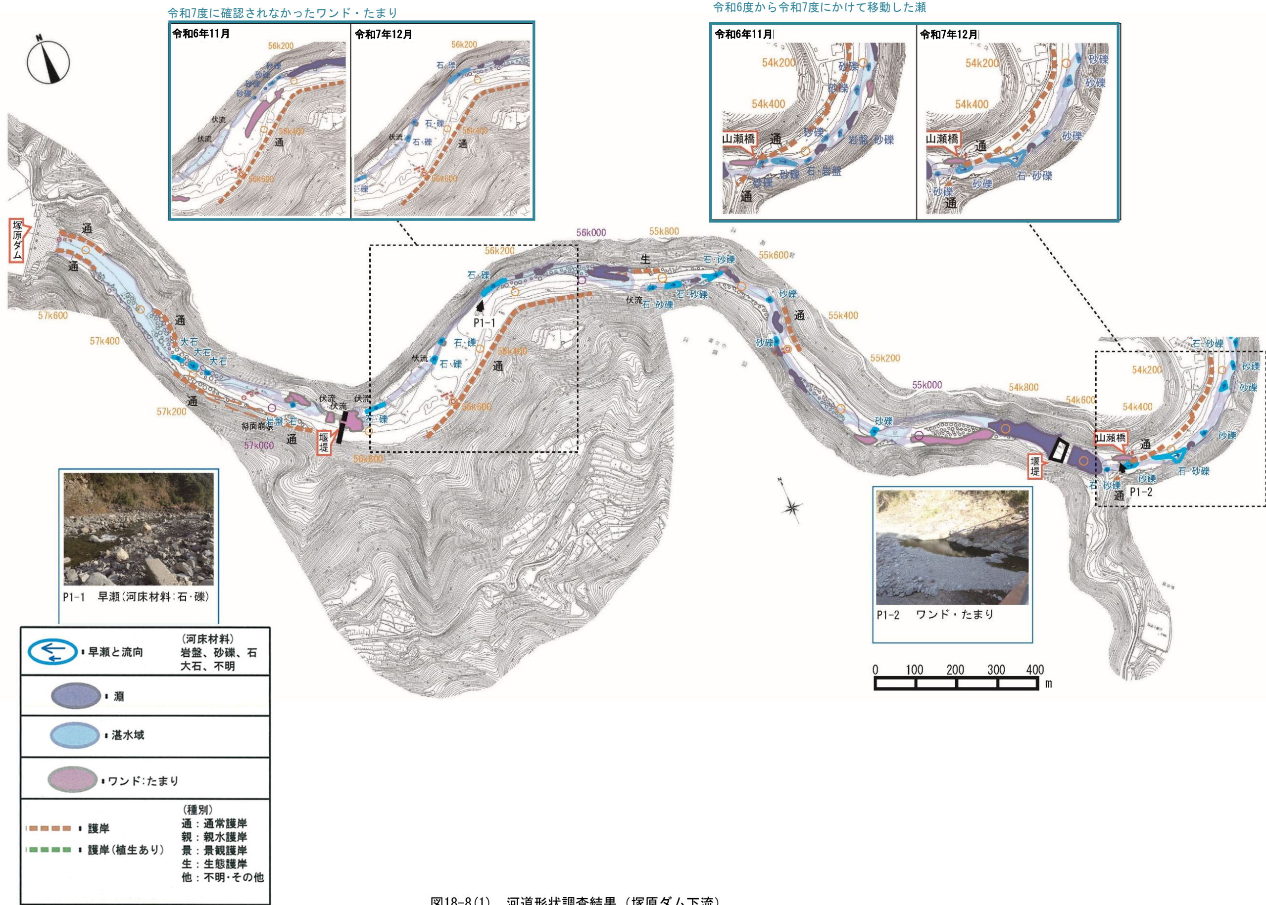
図18-8(1) 河道形状調査結果（塚原ダム下流）
