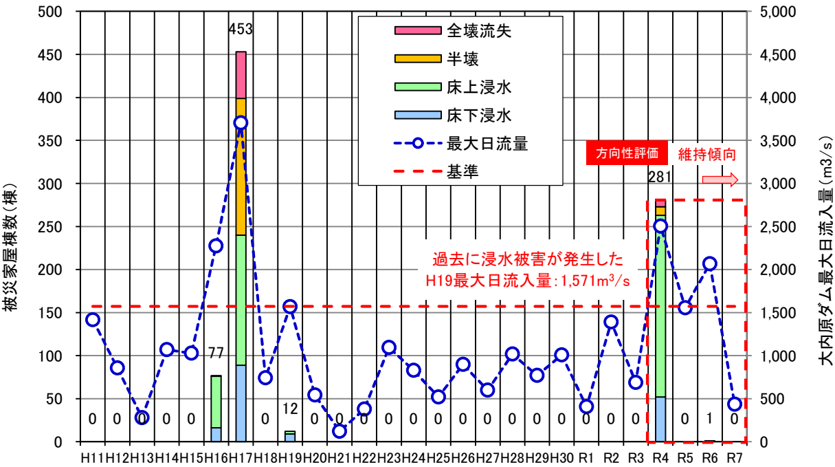
図24-1 浸水被害家屋棟数の推移 ※日流入量：毎正時流入量の24時間平均値 最大日流入量：日流入量の年間最大値 ※被害家屋棟数は支川の被害も含む
