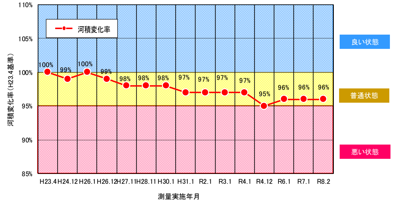
図23-1 河積変化率の経年変化
