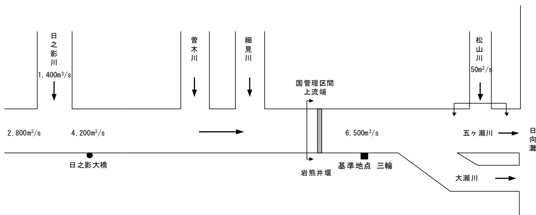
図 4-1 整備計画目標流量配分図
