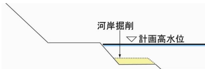
図 5-4 日之影地区五ヶ瀬川の河岸掘削概念図
