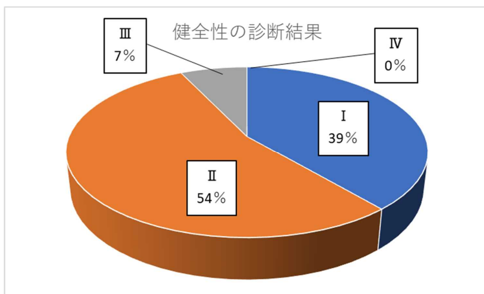
○点検に基づく健全性の診断結果（令和4年3月末時点）
