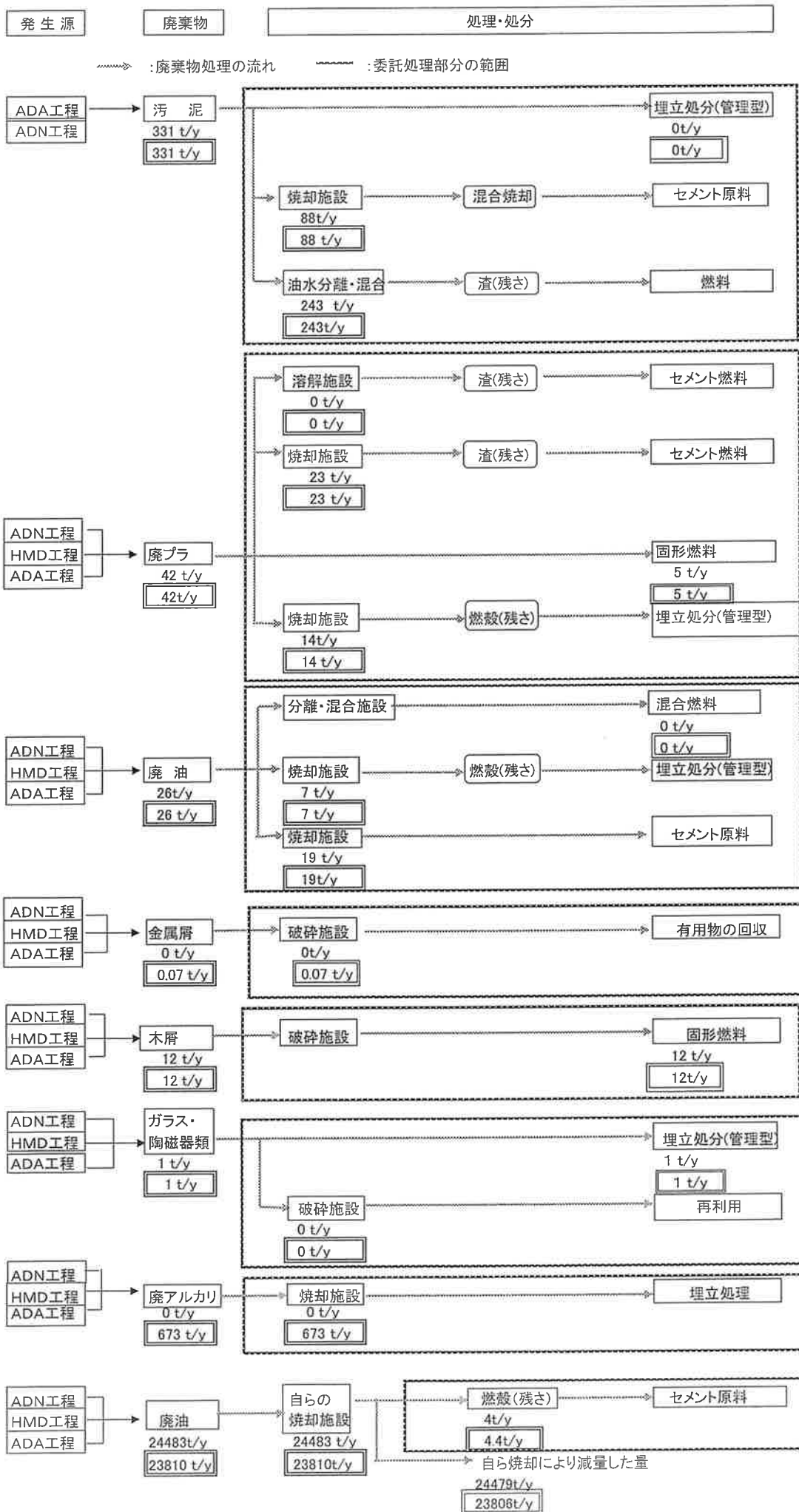
産業廃棄物処理フロー図(原料)
