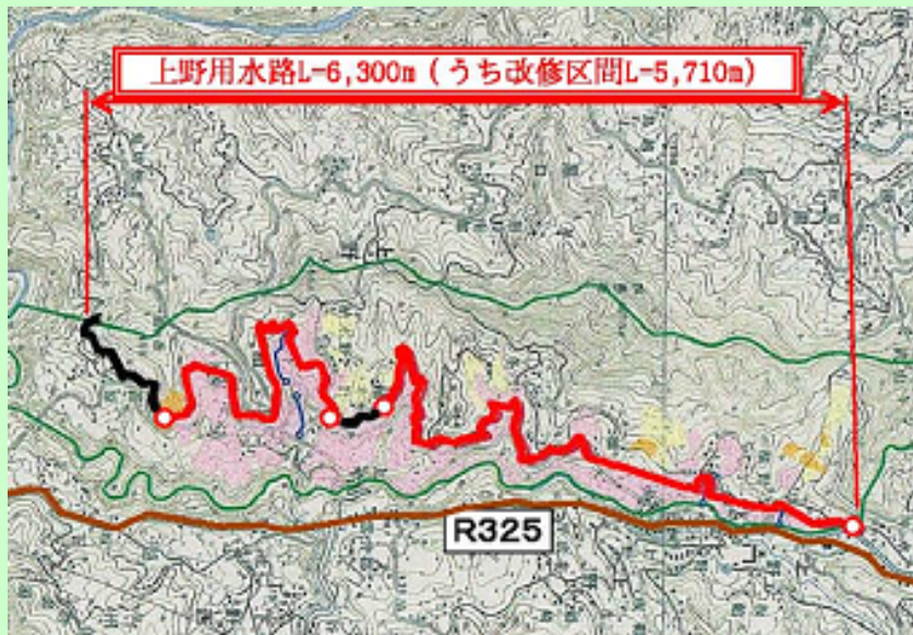
県営中山間地域総合農地防災事業 上野地区計画図
