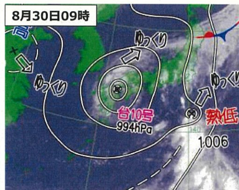
衛星画像（赤外）と地上天気図
