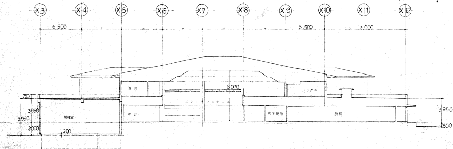
木筋鉄断面図
