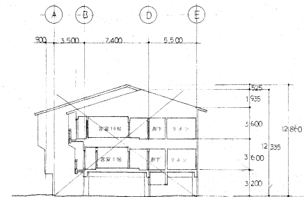
浴場棟断面図
