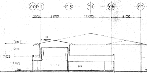
木筋鉄断面図
