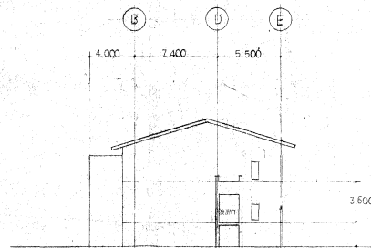
浴場下断面図
