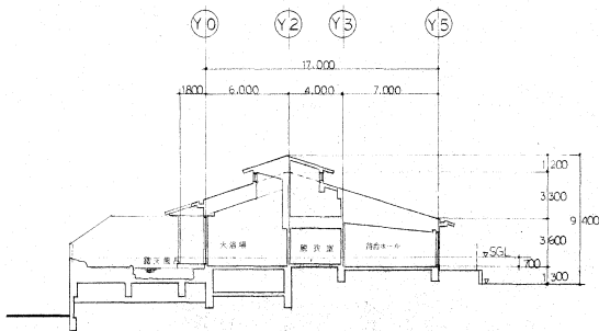
木浴場断面図
