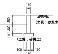
④号擁壁 S=1:50 (土留め小構造物) H=1.0m以下
