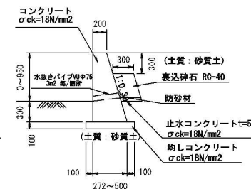
③号擁壁 S=1:50 (土留め小構造物) H=1.0m以下
