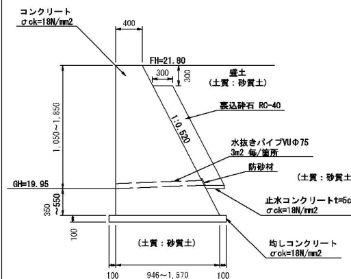
①号擁壁 S=1:50
