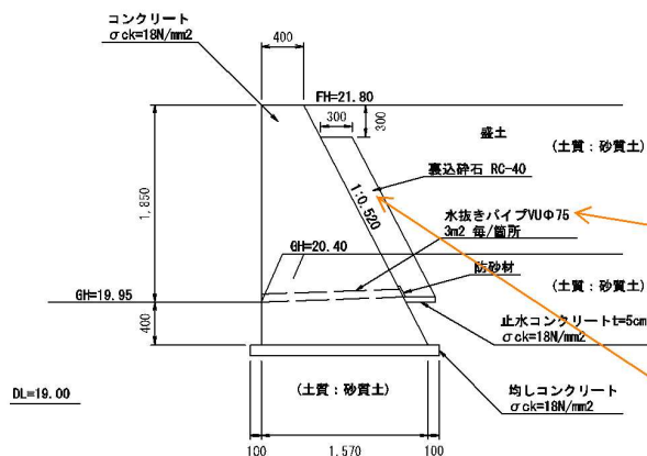
①-①断面図 S=1:50
