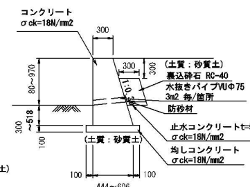
②号擁壁 S=1:50 (土留め小構造物) H=1.0m以下
