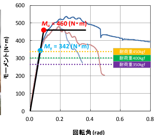
(2) モーメントー回転角の関係
