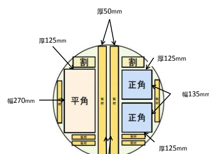
図 1 木取り
