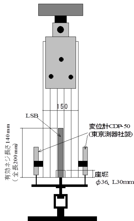
図2 試験方法の概要
