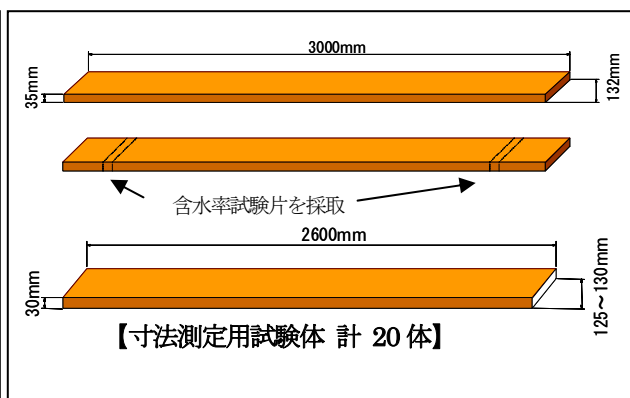
図2 Bグループ試験体作成概略図
