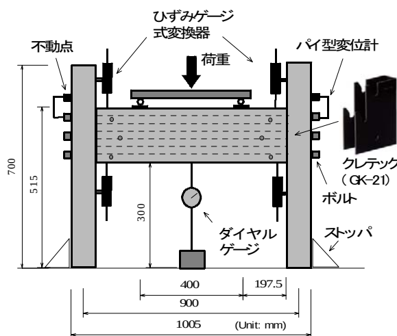
図1 柱-梁接合部せん断クリープ試験体
