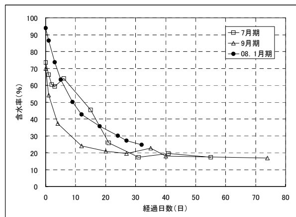
図 4 スギ板材天乾実験 平均含水率変動比較
