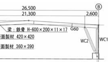
図3 ハイブリッド構法の構造面図
