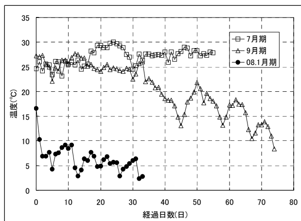
図 6 スギ板材天乾実験 実験期間平均気温比較
