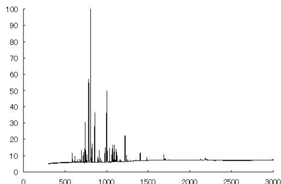
図2 中温乾燥により得られたスギ精油のクロマトグラム
