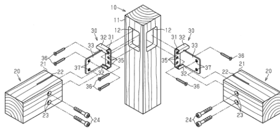
図 1 造作金具の外観と接合方法
